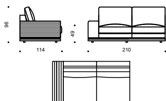
Модуль двухместный L/R/ модуль двухместный большой L/R L210 / 230 P114 H96
