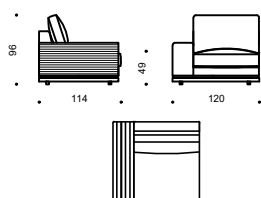
Модуль одноместный L/R/ Модуль одноместный большой L/R L120 / 130 P114 H96
