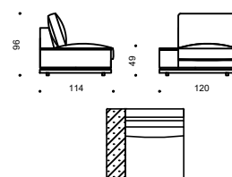
Модуль одноместный со столиком L/R/ Модуль одноместный со столиком большой L/R L120 / 130 P114 H96
