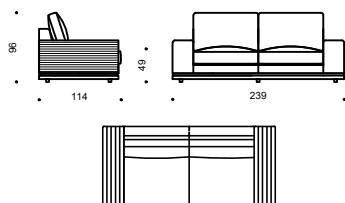
Диван/ Диван большой L239 / 259 P114 H96
