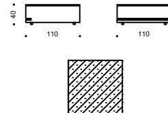
Угловой модуль со столиком L/R L110 P110 H40
