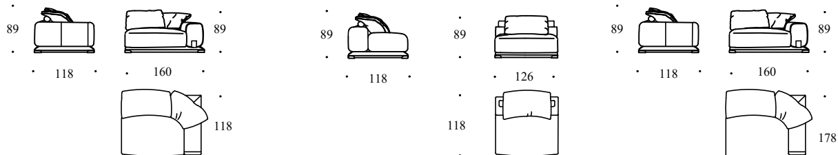
Модуль центральный
