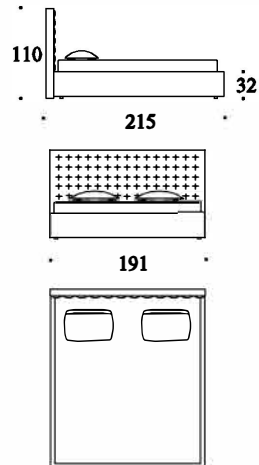
Кровать L 191 P 215 H 110
