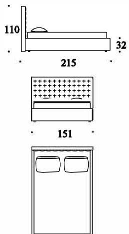
Кровать L 151 P 215 H 110
